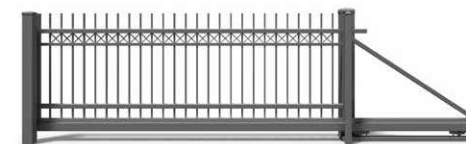
BRAMA PRZESUWNA TOP Maksymalna dostępna szerokość: 6000 mm Minimalna standardowa szerokość: 3000 mm Lewostronna oraz prawostronna
