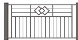
PRZEŚŁO PROSTE (TYP P) Maksymalna dostępna szerokość: 3000 mm Minimalna standardowa szerokość: 2000 mm
