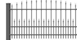
PRZĘSŁO WYPUKŁE (TYP W) Maksymalna dostępna szerokość: 3000 mm Minimalna standardowa szerokość: 2000 mm
